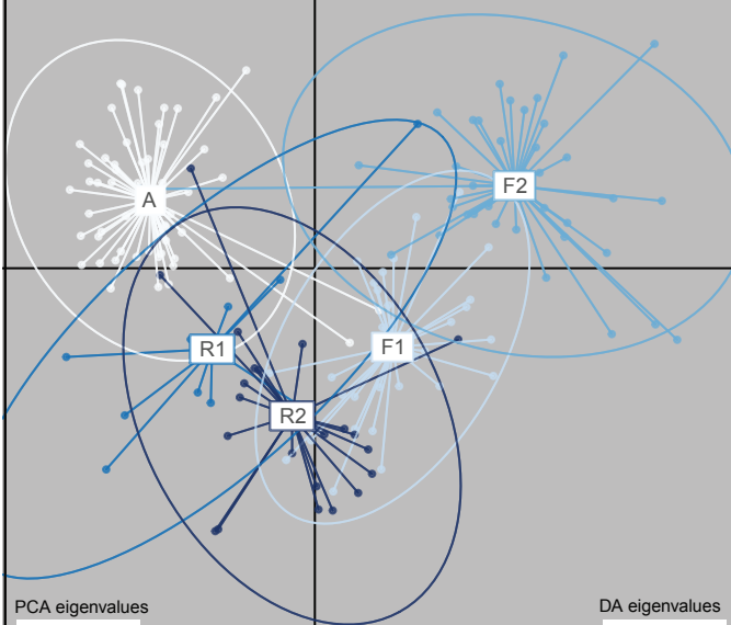
PCA eigenvalues
